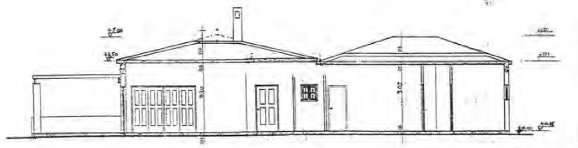
ΣΧΗΜΑΤΙΚΗ ΤΟΜΗ Α-Α
