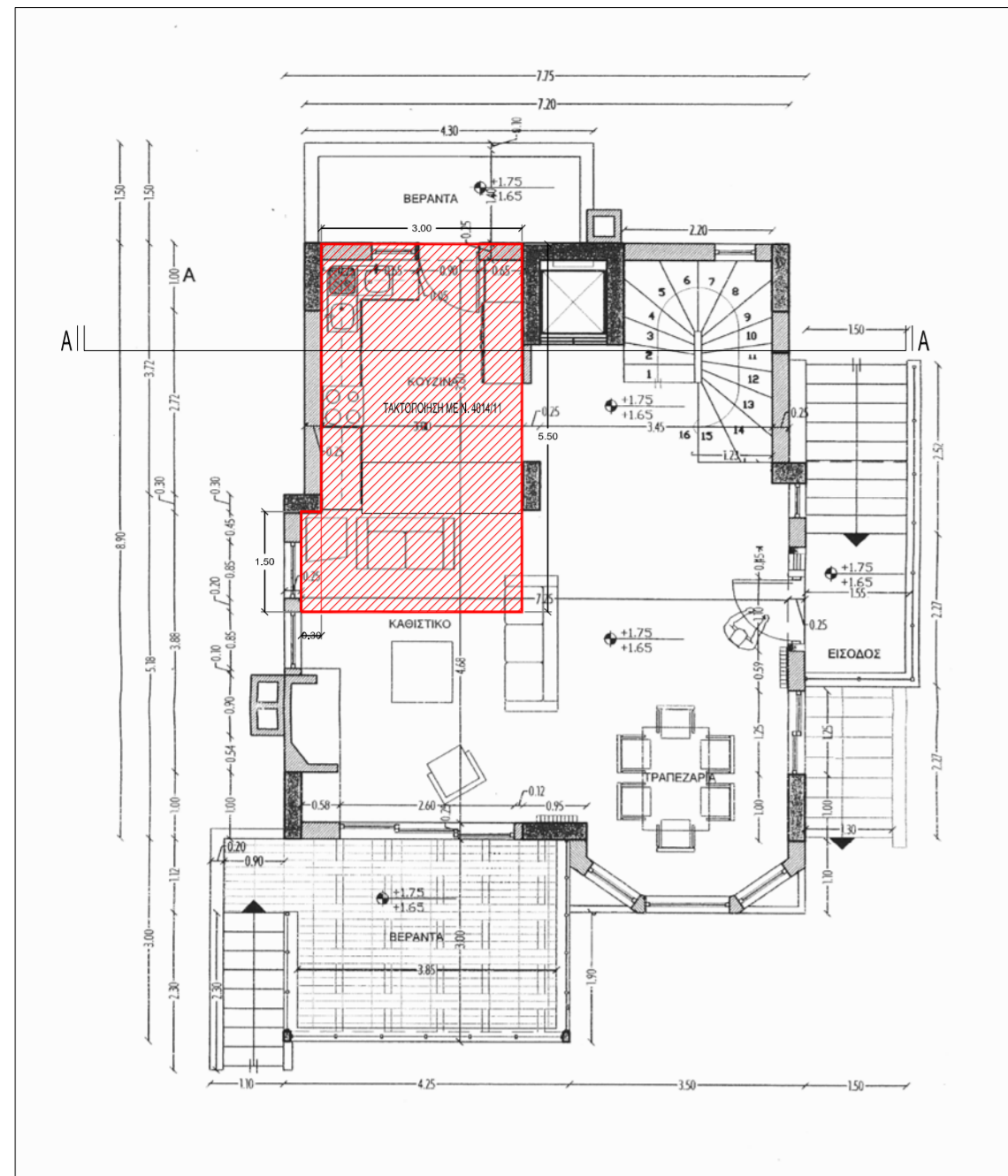
ΚΑΤΟΨΗ ΙΣΟΓΕΙΟΥ - ΑΠΟΤΥΠΩΣΗ
